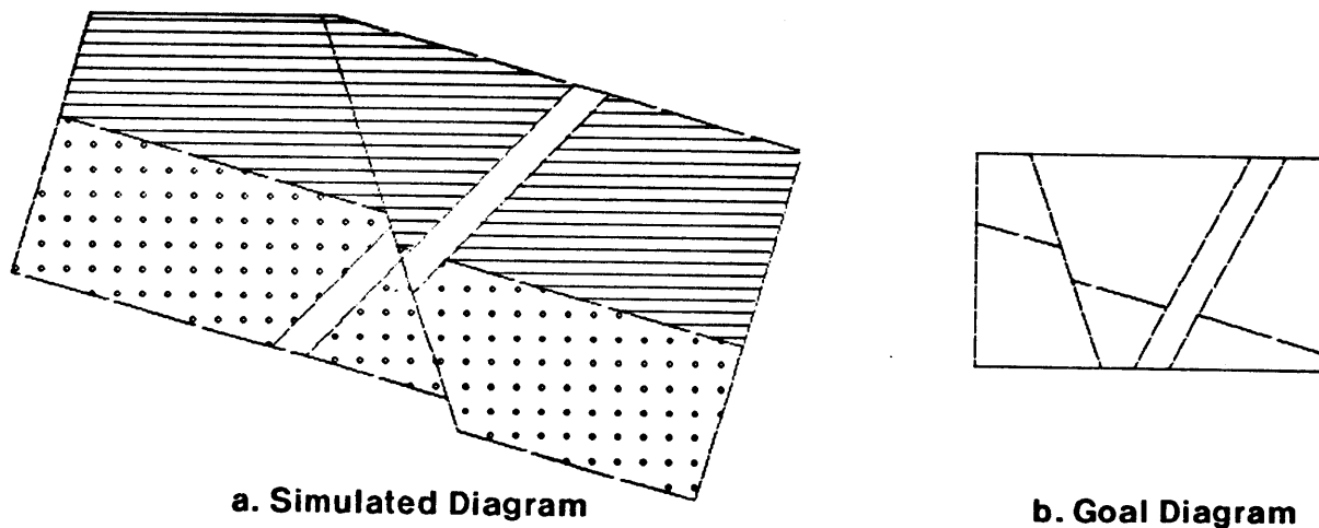
Fig. 7. Simulation Using Uncorrected Parameter Values
